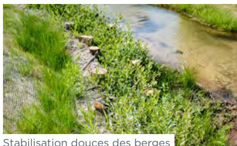
Stabilisation douce des berges
